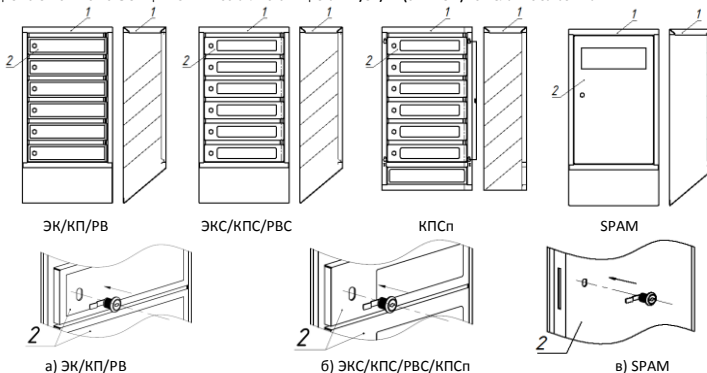
Рис. 1. Схема расположения и схема сборки Почтовых ящиков.
